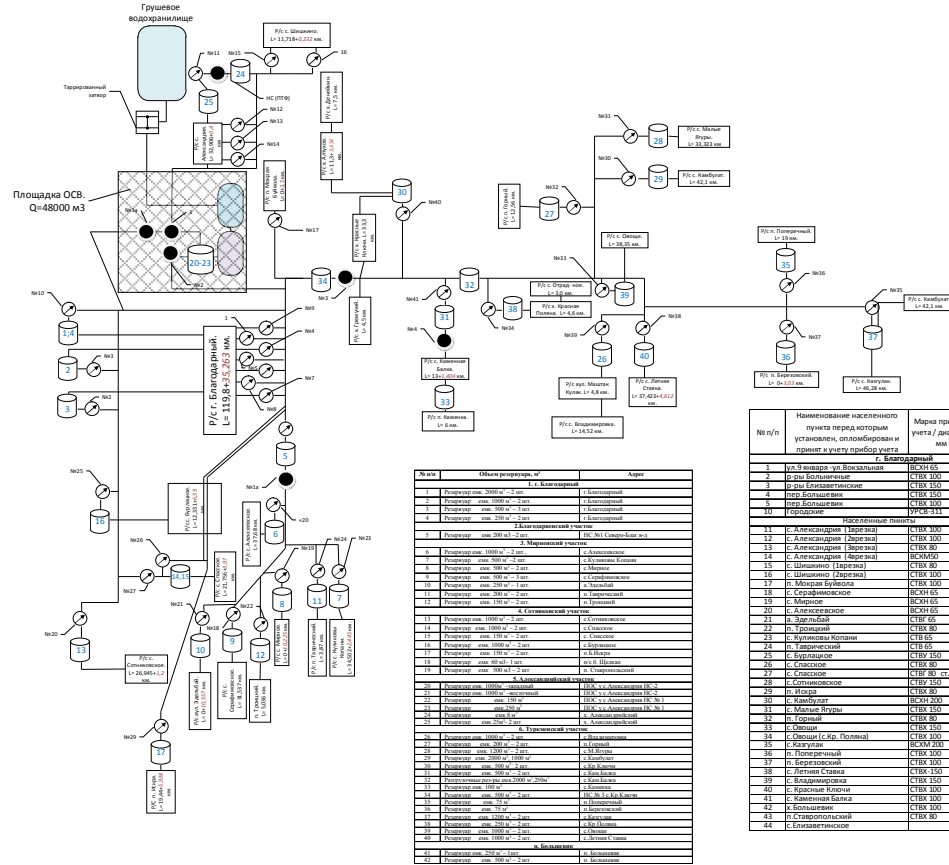
Схема водоснабжения филиала ГУП СК «Ставрополькрайводоканал» Благодарненский «Межрайводоканал».
